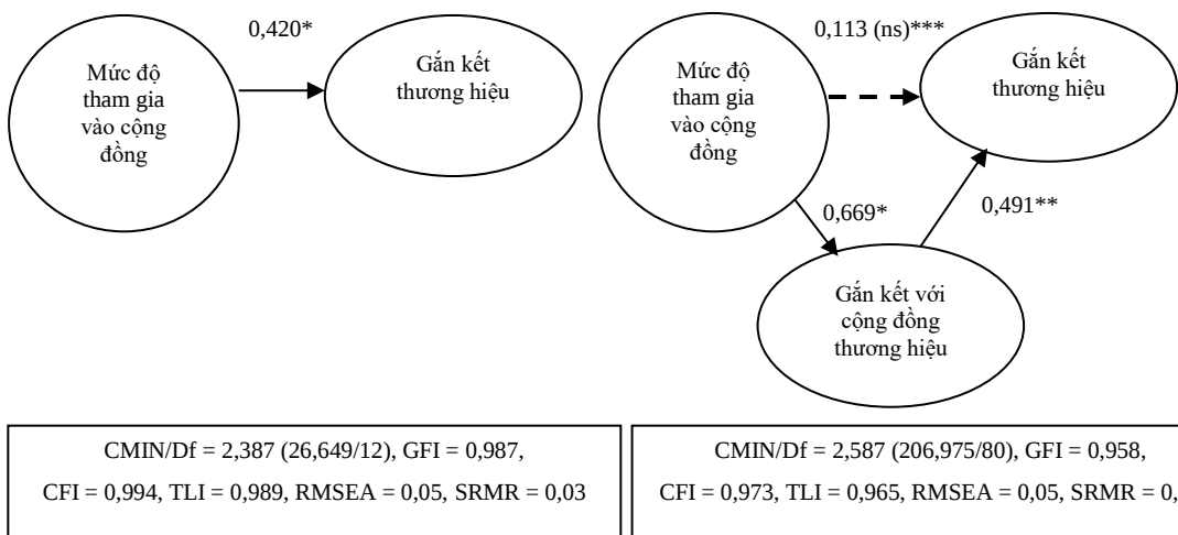
Hình 3. Hai mô hình cấu trúc tuyến tính kiểm định giả thuyết H1
